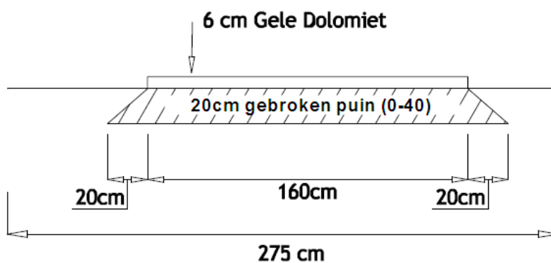
Doorsnede van een aangelegd pad
